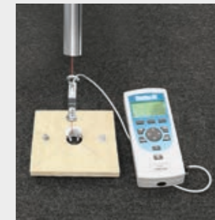
Testování pevnosti fixačních elementů
