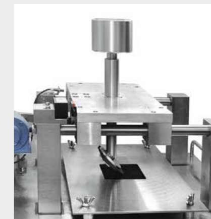
Přístroj na provádění podpatkového testu
