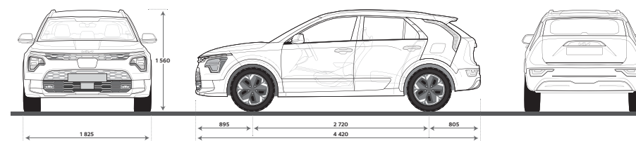
Rozměry verze EV (mm)
