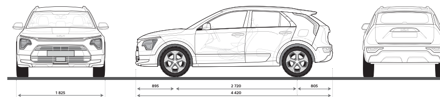
Rozměry verzí HEV/PHEV (mm)
